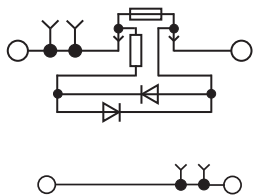
Электрическая схема рис. 1
