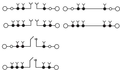
Электрическая схема рис. 1
