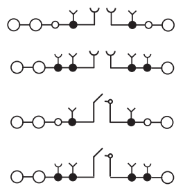
Электрическая схема рис. 1
