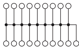
Электрическая схема рис. 1
