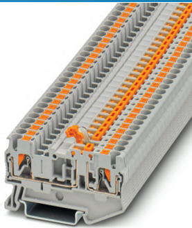
Рис. 1 2 контакта с ножевым размыкателем
