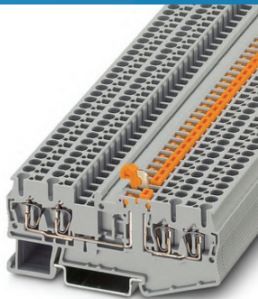
Рис. 1 4 контакта с ножевым размыкателем
